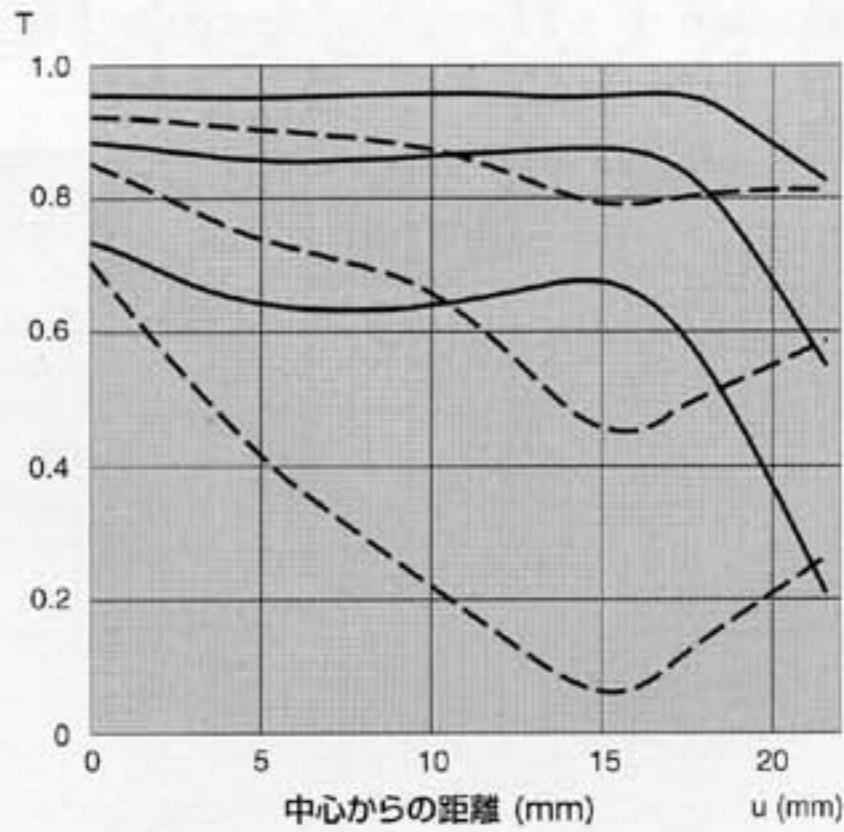
図2 MTF (F8)
